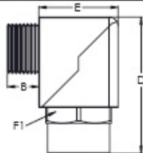
EM - Elbow
